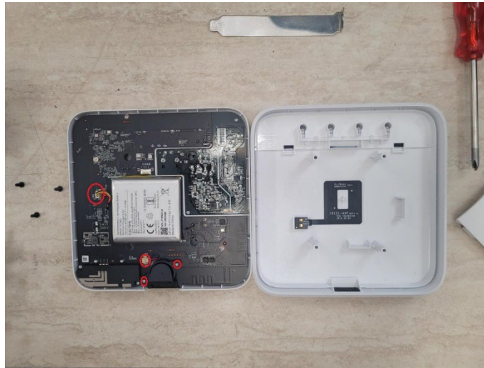
3. ábra Az eszköz alján található hangszóró és az azt rögzítő csavarok
